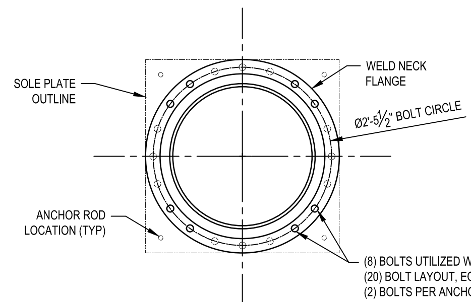
B DETAIL - FLANGE SCALE: 3/4" = 1'-0"
